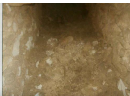
Portion B – PM5 – Dépôts en radier (blocs de maçonnerie) probablement issues de chutes
